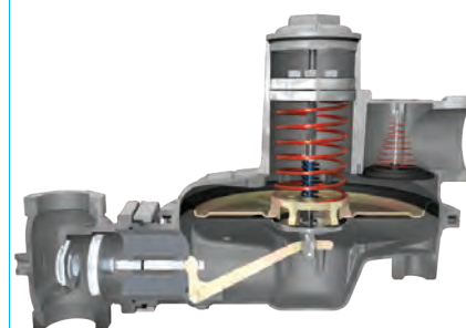
WIDOK WEWNĘTRZNY TYP CS800
