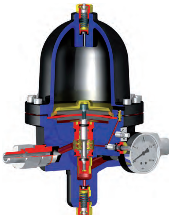
PRZEKRÓJ URZĄDZENIA TYPU RP/10
