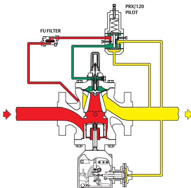
TYP EZR-OS2 SCHEMAT DZIAŁANIA
