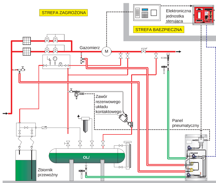
PRZYKŁAD INSTALACJI TYPU OL/ W KOMPLETNYM SYSTEMIE NAWANIAJĄCYM Z DOSAODOR-D
