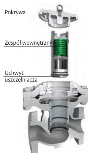
OPATENTOWANE DLA DN 100 SYSTEM ŁATWEJ OBSŁUGI
