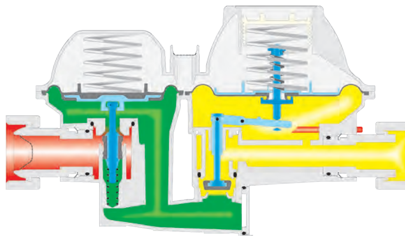
TYP B NG SCHEMAT DZIAŁANIA
