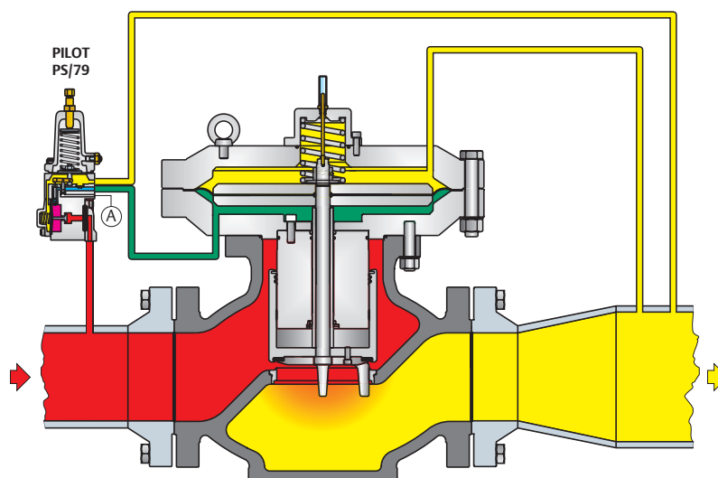
TYP 971 SCHEMAT DZIAŁANIA
