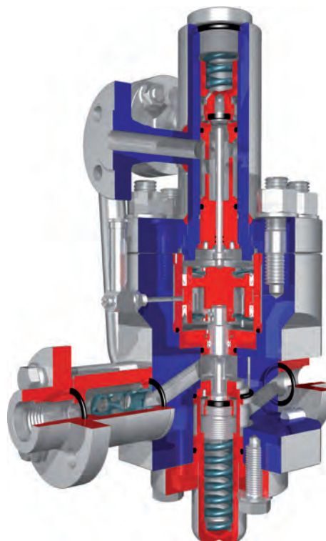
PRZEKRÓJ URZĄDZENIA TYPU RLC/20
